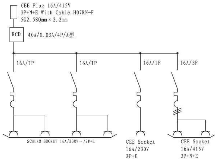
Bloková schéma elektrického zapojenia
