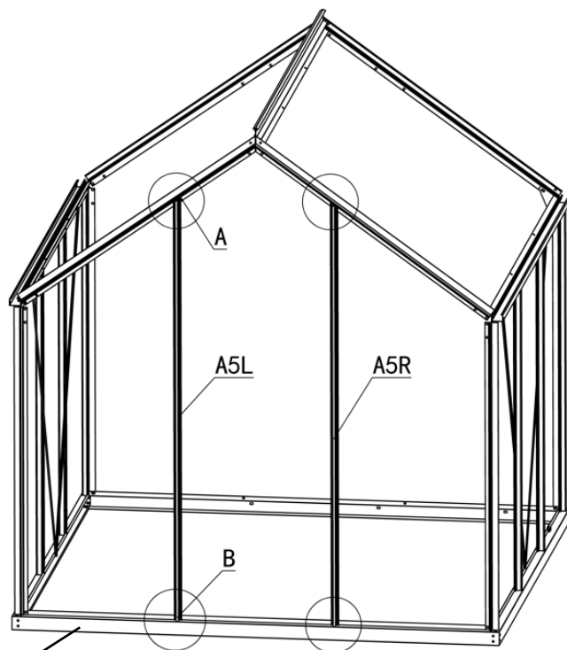
Zadný pohľad
