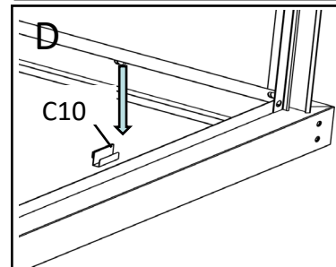
Pohľad zľava
