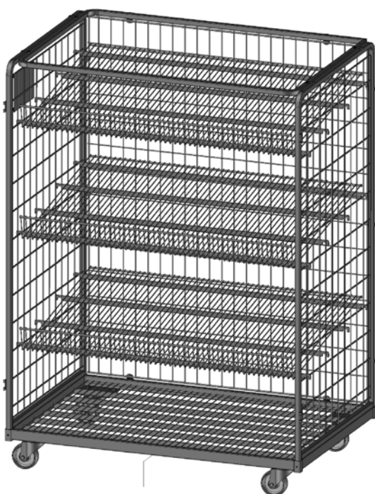
Obr. 8 Model so zadnou stenou a šikmo umiestnenými policami so zdvihnutými hranami
