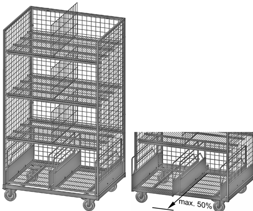
Obr. 11 Model so zásuvkami
