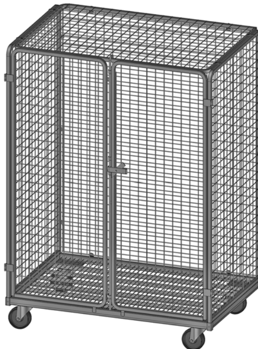
Obr. 10 Model s mriežkovým vekom a dvermi
