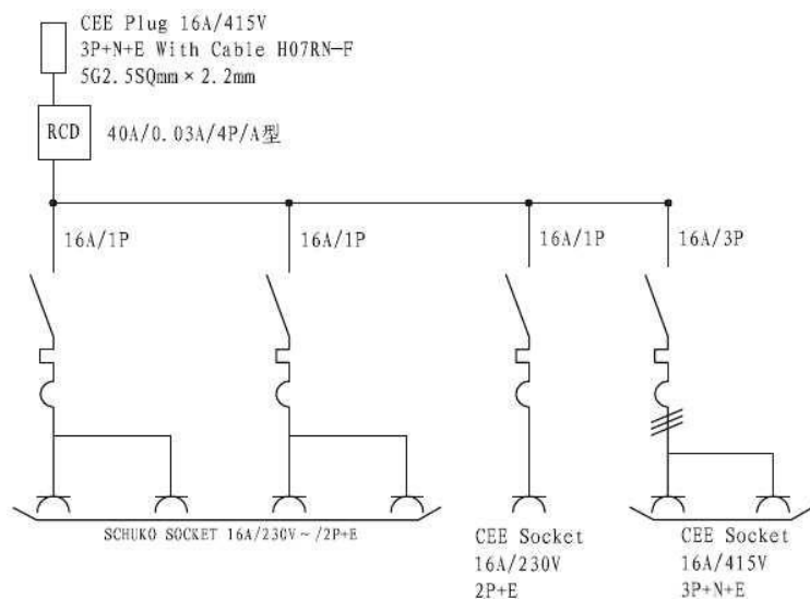
Bloková schéma elektrického zapojenia
